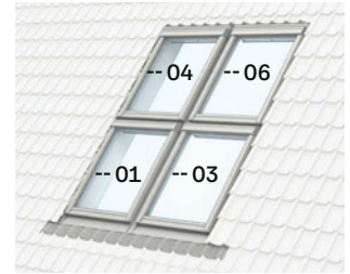
Üst üste ve yan yana kombinasyon
